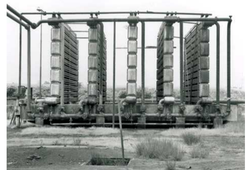
9) Rieselkühler
